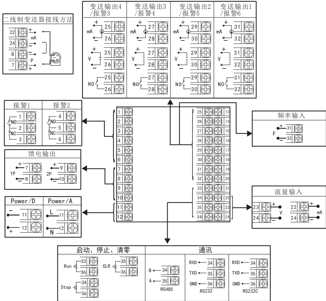
OHR-G601/G601R系列接线图
