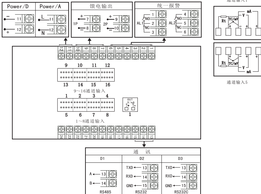
A、B型统一变送接线图
