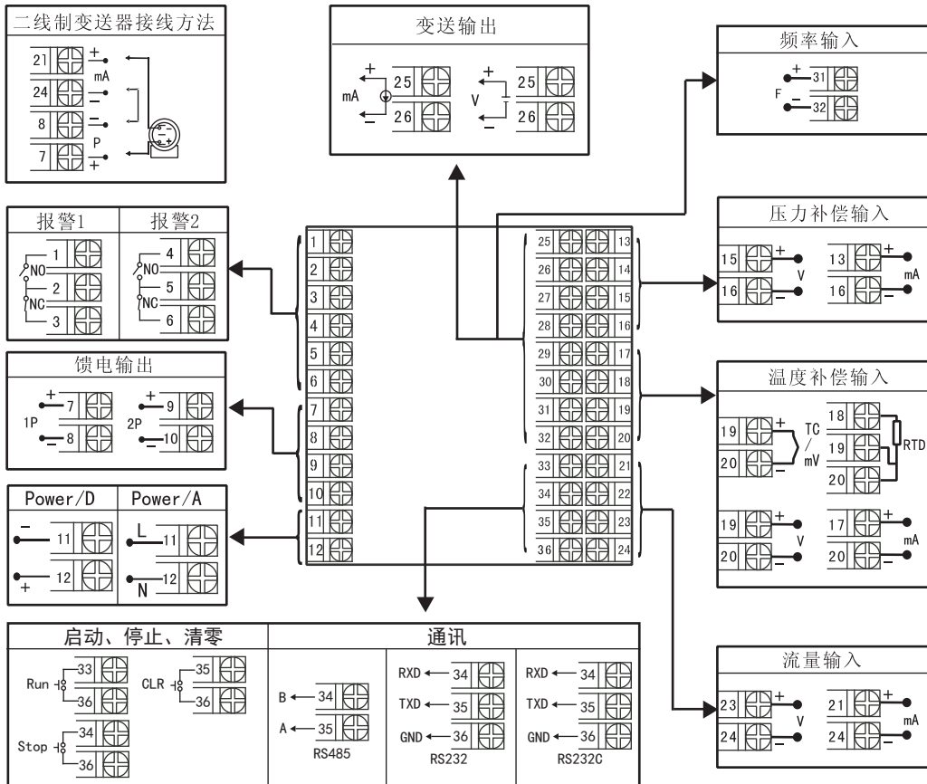
OHR-F602R接线图
